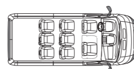
Panorama tengelytáv 3450 mm 8/9 személyes
